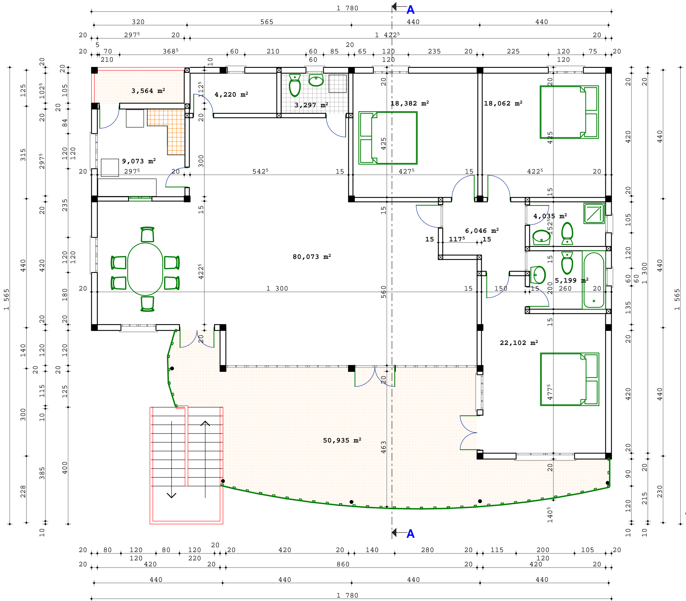
VUE EN PLAN DU R+1
